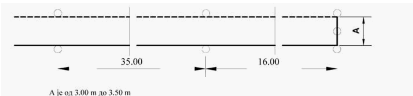
Slika 28. Prostor i oznake prostora za izvođenje poligonske radnje "kočenje i zaustavljanje" (za osposobljavanje kandidata za vozače motornih vozila kategorije M)
