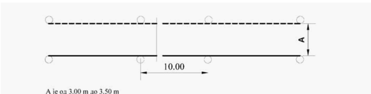
Slika 27. Prostor i oznake prostora za izvođenje poligonske radnje "vožnja napred sa promenom stepena prenosa i unazad u istoj saobraćajnoj traci" (za osposobljavanje kandidata za vozače motornih vozila kategorije M)
