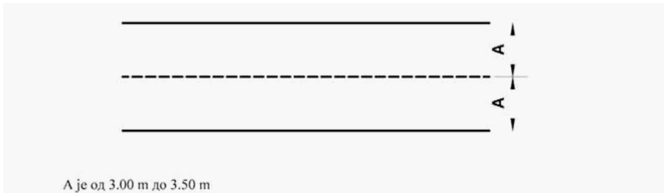
Slika 11. Prostor i oznake prostora za izvođenje poligonske radnje "odvajanje i spajanje vučnog i priključnog vozila" (za osposobljavanje kandidata za vozače vozila kategorije BE)
