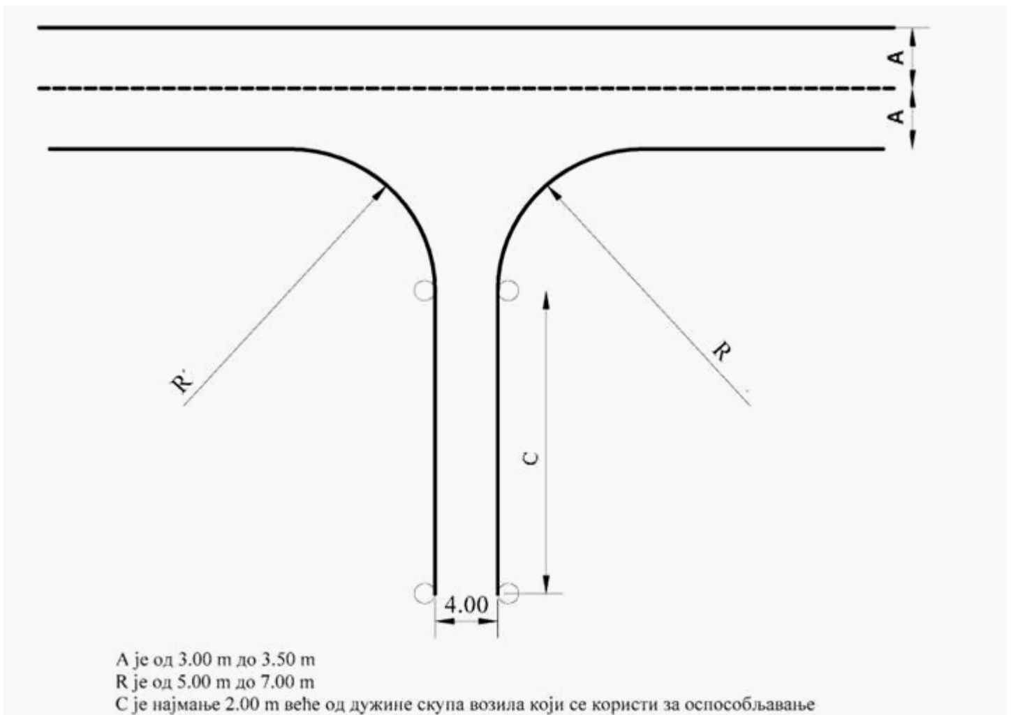
Slika 13. Prostor i oznake prostora za izvođenje poligonske radnje "voжnja unazad sa skretanjem ulevo, odnosno udesno, pod pravim uglom" (za osposoblјavanje kandidata za vozače vozila kategorije BE)
