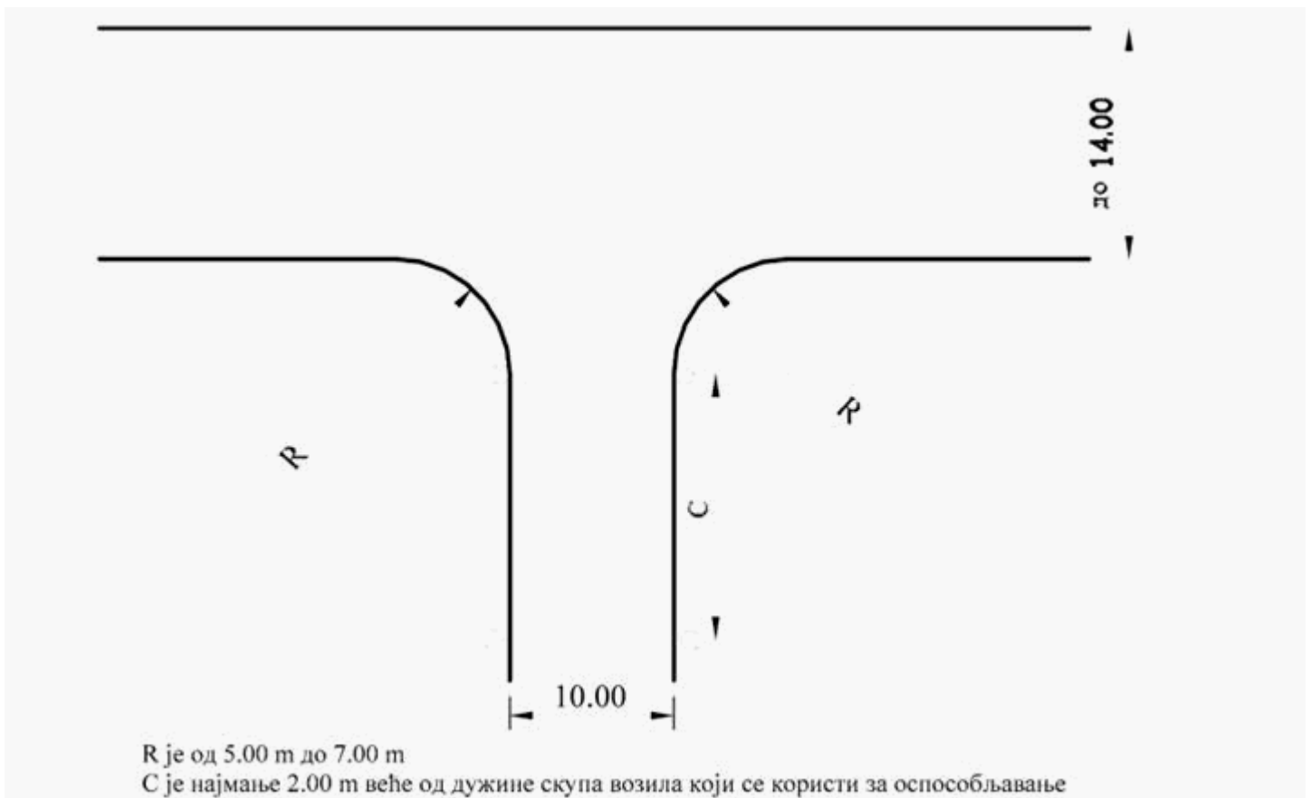
Slika 23. Prostor i oznake prostora za izvođenje poligonske radnje "vožnja unazad sa skretanjem ulevo, odnosno udesno, pod pravim uglom" (za osposobljavanje kandidata za vozače vozila kategorija D1E i DE)
