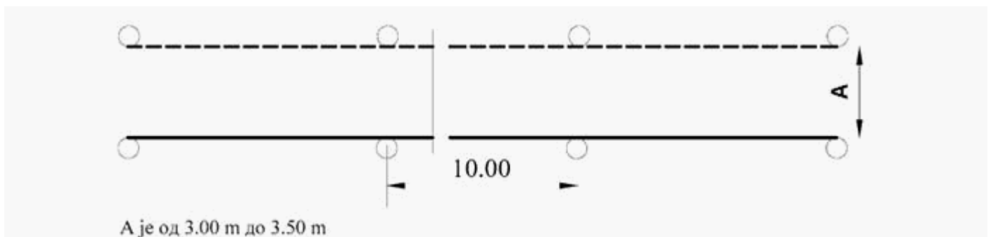
Slika 25. Prostor i oznake prostora za izvođenje poligonske radnje "vožnja napred sa promenom stepena prenosa i unazad u istoj saobraćajnoj traci" (za osposobljavanje kandidata za vozače vozila kategorije F)
