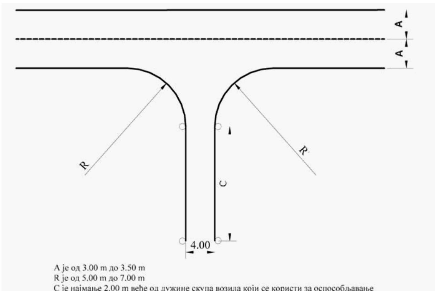
Slika 26. Prostor i oznake prostora za izvođenje poligonske radnje "vožnja unazad sa skretanjem ulevo, odnosno udesno, pod pravim uglom" (za osposobljavanje kandidata za vozače vozila kategorije F)
