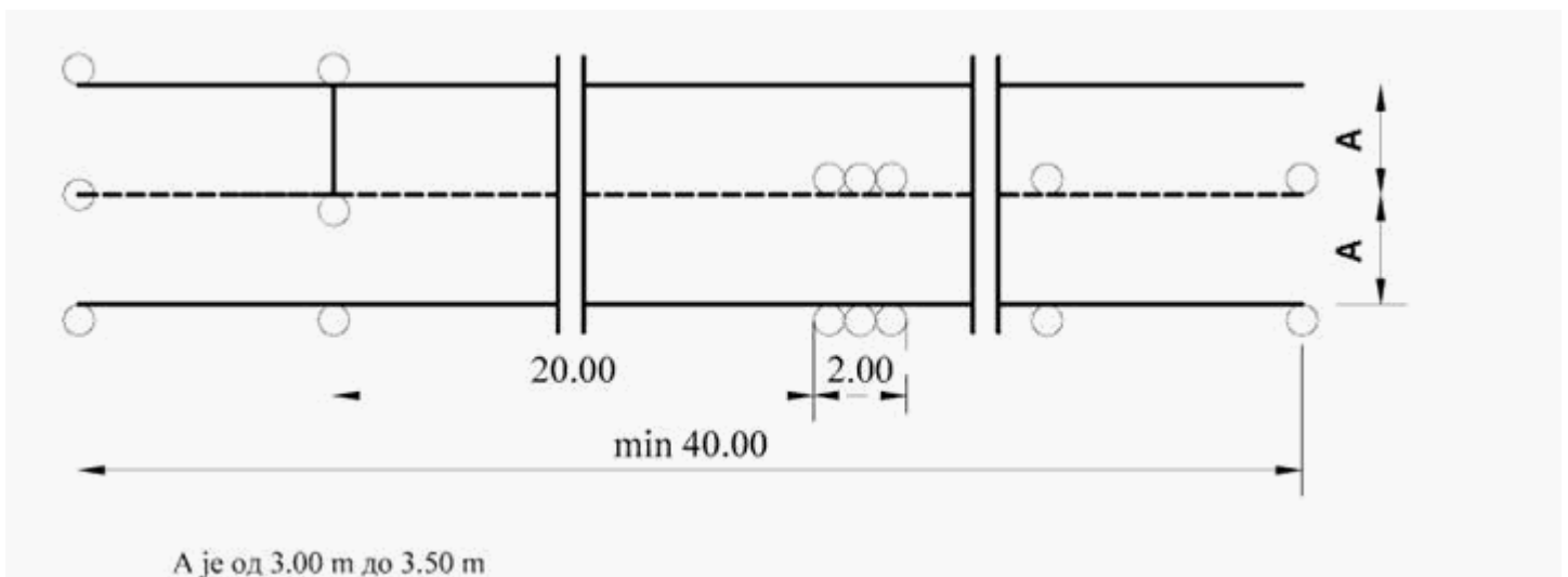
Slika 14. Prostor i oznake prostora za izvođenje poligonske radnje "voжnja napred sa promenom stepena prenosa i unazad sa promenom saobraćajne trake" (za osposoblјavanje kandidata za vozače motornih vozila kategorija C1 i C)
