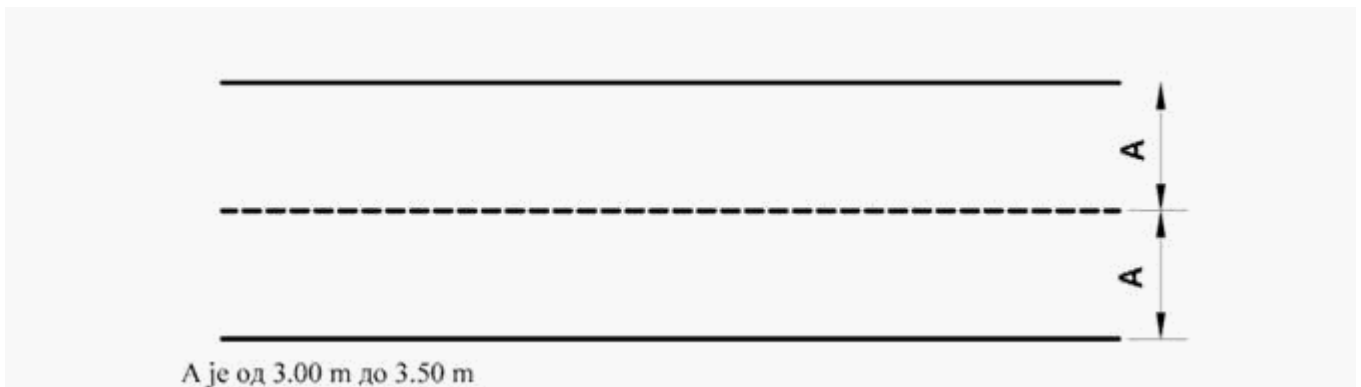
Slika 24. Prostor i oznake prostora za izvođenje poligonske radnje "odvajanje i spajanje vučnog i priključnog vozila" (za osposobljavanje kandidata za vozače vozila kategorije F)
